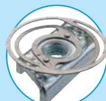
140-02 Dado rapido pesante
